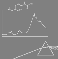
IR/NIR-Spektroskopie
